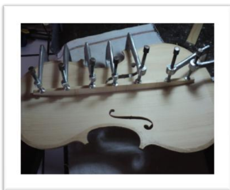
Ilustración 6. Barra armónica
